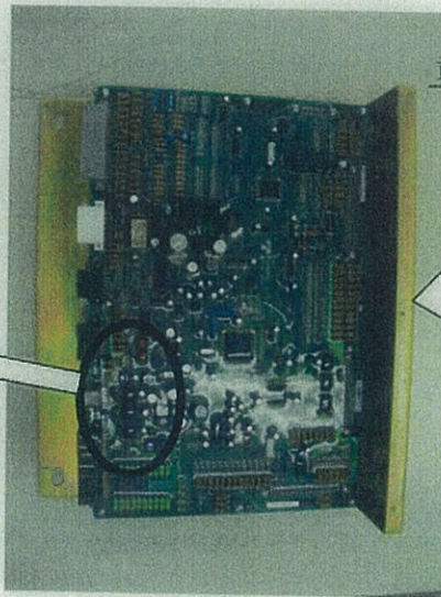
多重送電ユニット内基板
